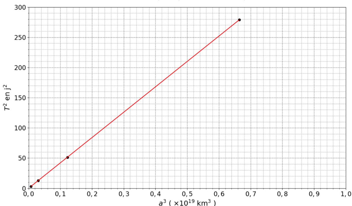
Figure 1. T^2 en fonction de a^3 .
